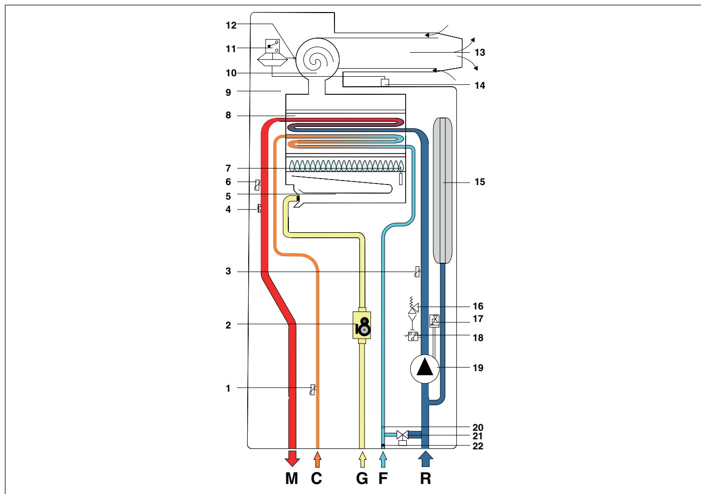
Fig. 5 Esquema hidráulico CTFS
