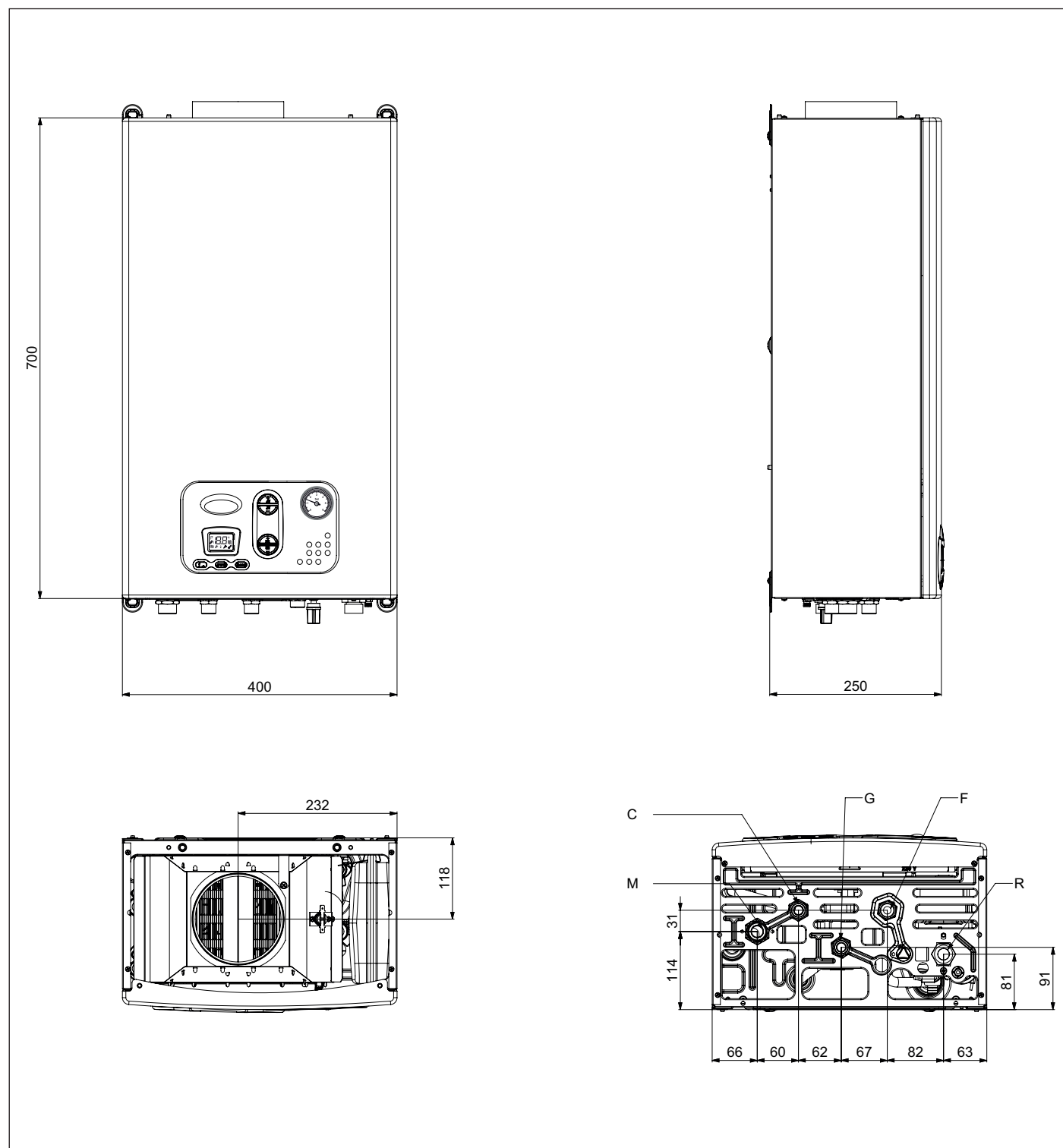
Fig. 4 Dimensiones CTN
