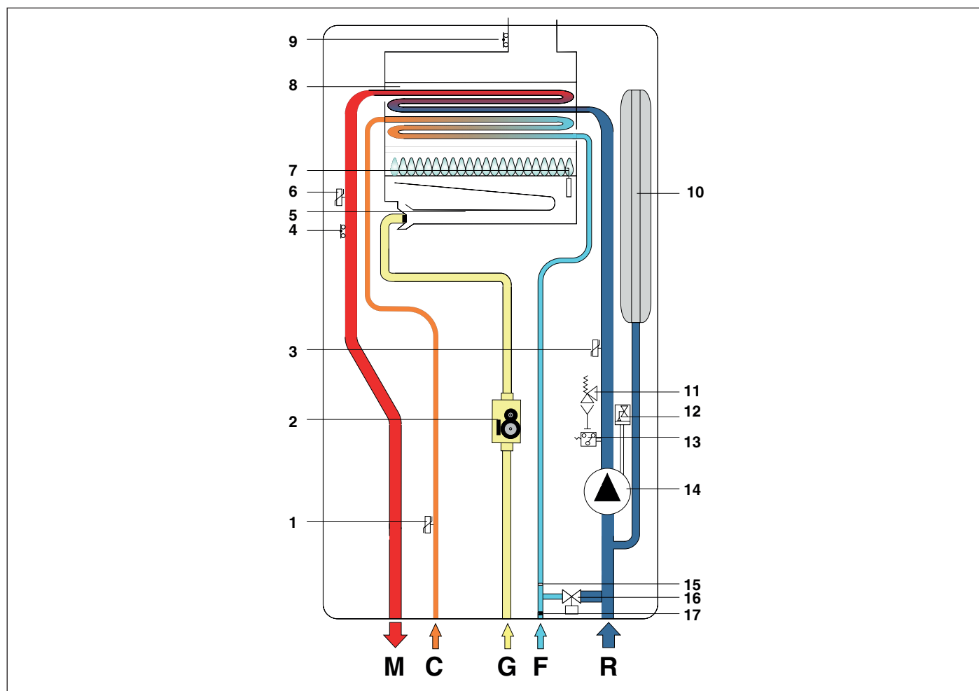
Fig. 6 Esquema hidráulico CTN
