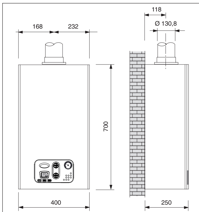
Fig. 9 Cotas dimensionales para la conexión al conducto de evacuación de humos de los modelos con cámara abierta
