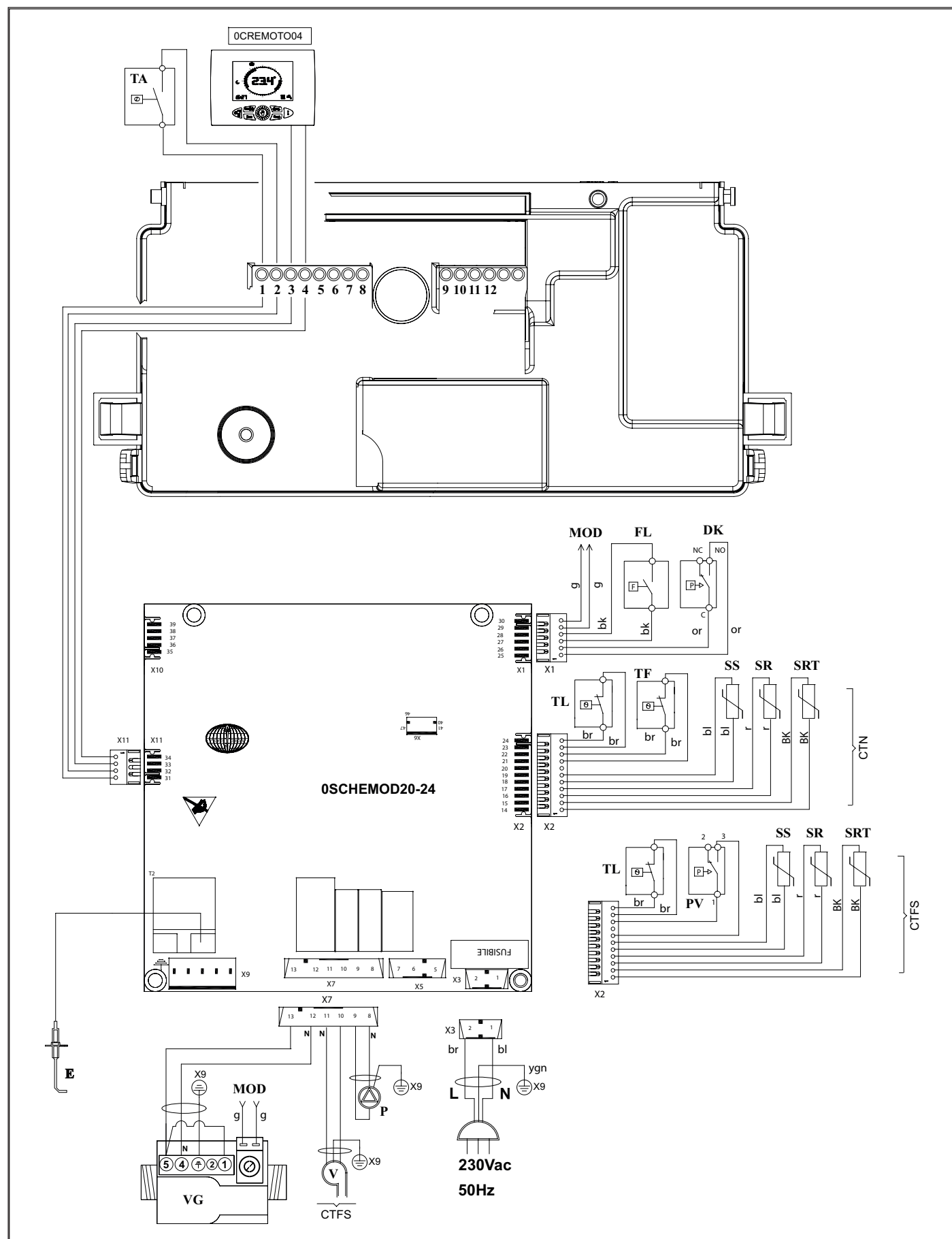
Fig. 20 Esquema eléctrico
