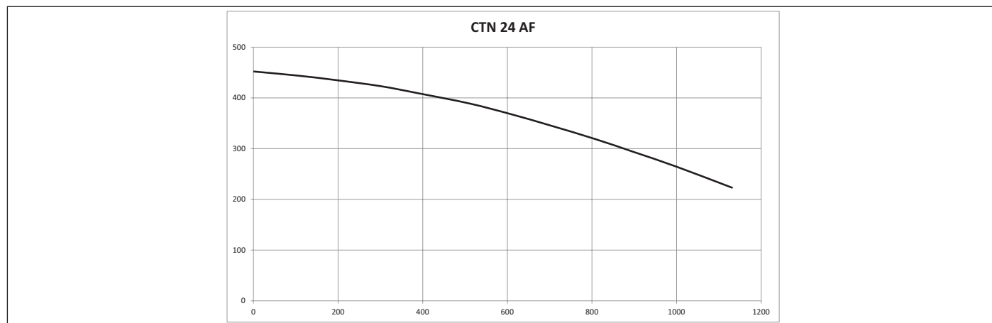
Fig. 19 Prevalencia disponible CTN 24 AF
