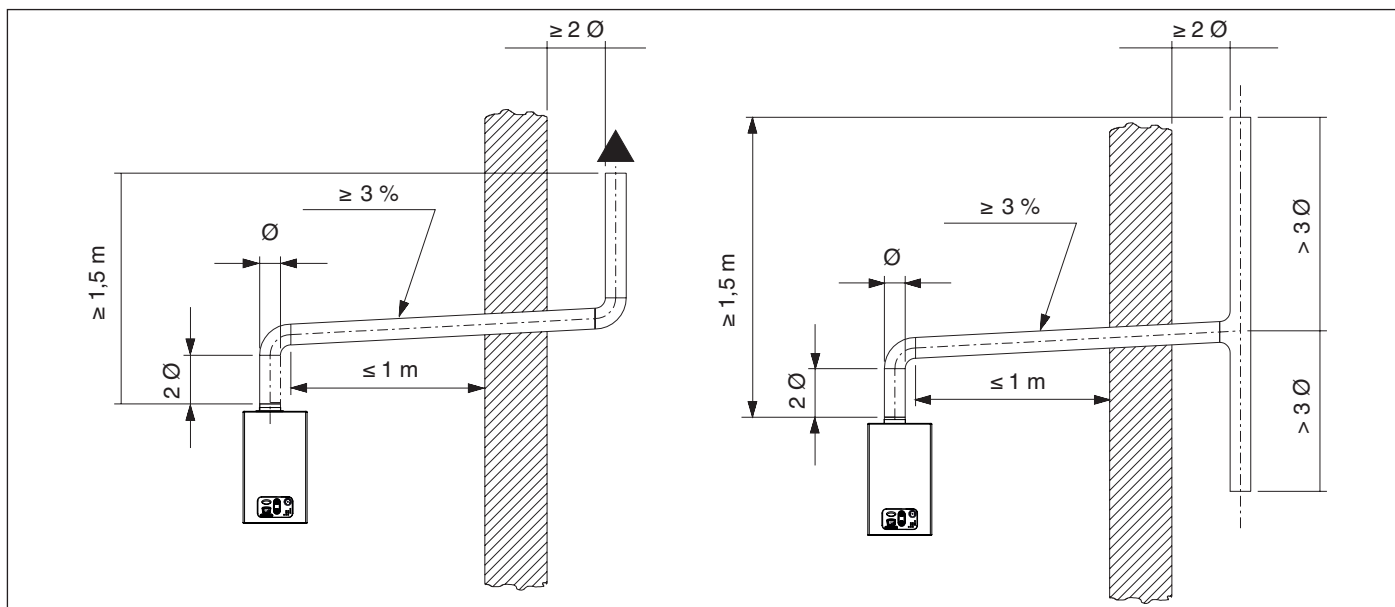
Fig. 8 Conexiones a los conductos de aspiración aire/evacuación de humos de los modelos de cámara abierta.
