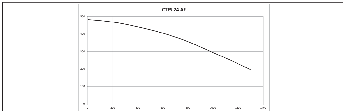
Fig. 18 Prevalencia disponible CTFS 24 AF
