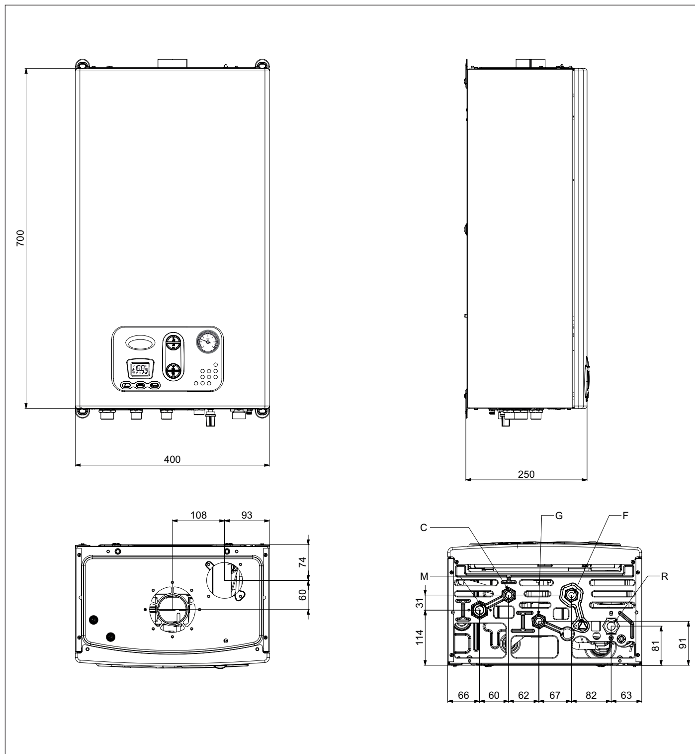
Fig. 3 Dimensiones CTFS
